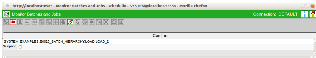
Abbildung 21.8: Confirm Maske
